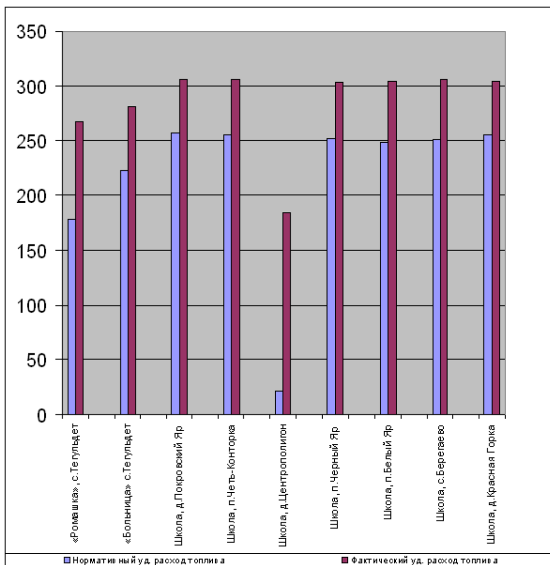
Рис. 3.1. Сравнение нормативных и фактических удельных расходов топлива на котельных Тегульдетского района
