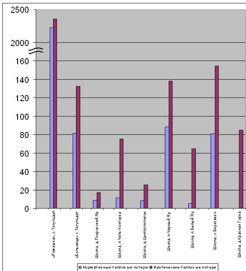
Рис. 3.2. Сравнение нормативных и фактических тепловых потерь на котельных Тегульдетского района
